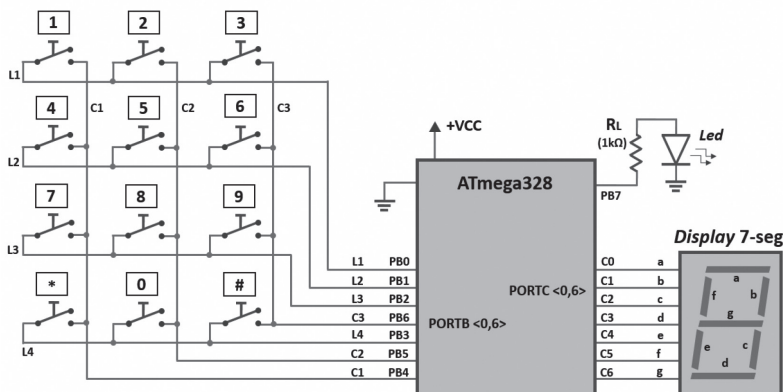
Figura 3.23 | Circuito como solução para a situação-problema
