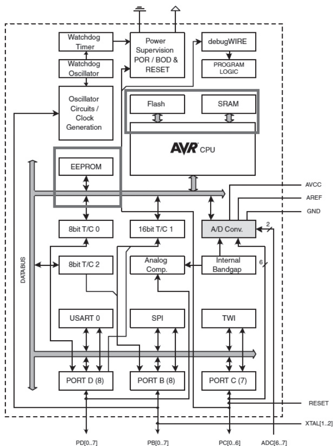
Figura 4.21 | Disposição das memórias no Microcontrolador ATmega328
