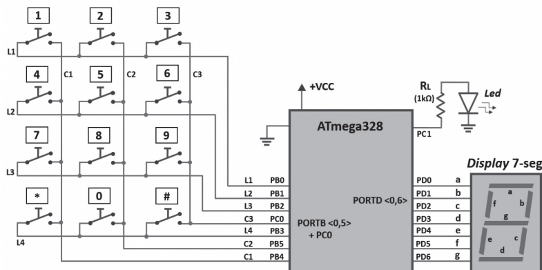
Figura 3.14 | Proposta de hardware para solução do problema
