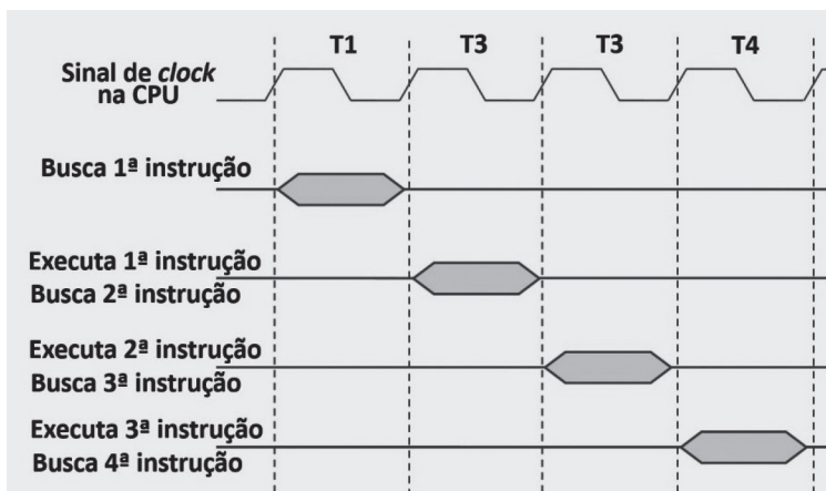
Figura 1.10 | Execução das primeiras instruções em pipeline
