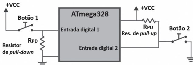
Figura 3.3 | Entradas digitais com resistores de pull-down e pull-up
