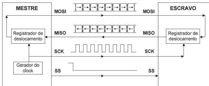
Figura 4.15 | Conexão Mestre-Escravo no protocolo SPI
