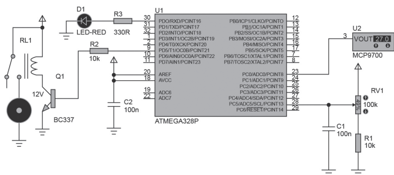
Figura 4.8 | Diagrama de hardware
