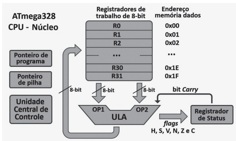
Figura 1.6 | Núcleo do ATmega328
