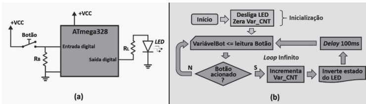
Figura 1.17 | (a) Circuito; (b) fluxograma/algoritmo para o exemplo
