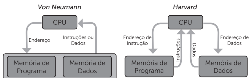
Figura 1.2 | Arquiteturas de computador Von Neumann e Harvard
