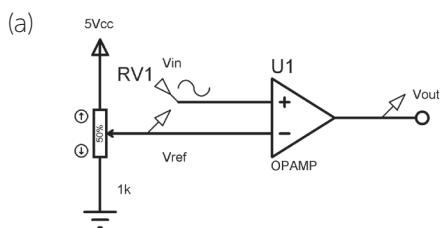
Figura 4.3 | Conversor analógico-digital de 1 bit: (a) esquemático de circuitos (b) onda resultante em Vout
