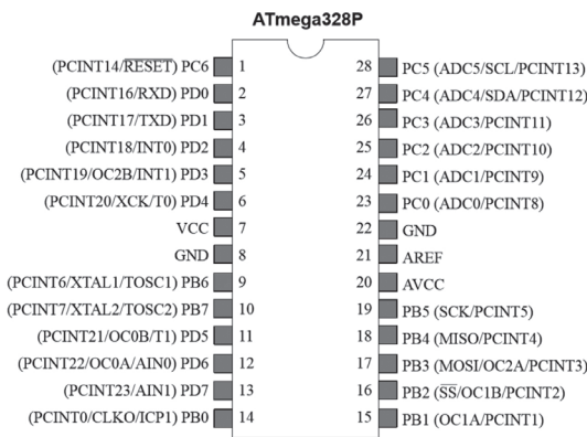
Figura 3.1 | Identificação e mapeamento das portas digitais nos pinos do ATmega328P
