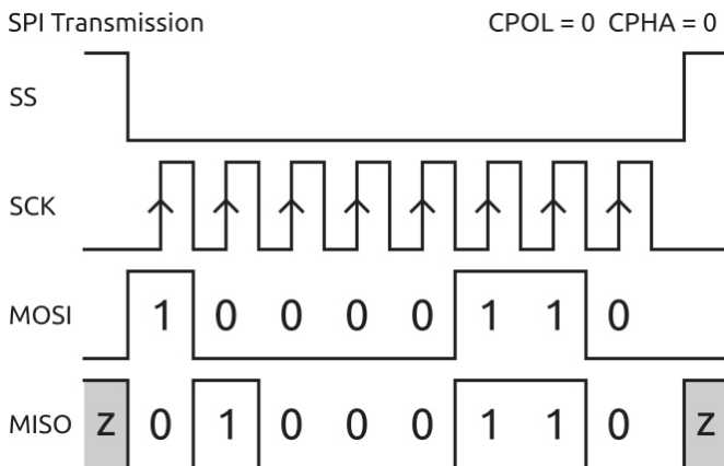
Figura 4.12 | Transferência síncrona SPI do valor 10001100
