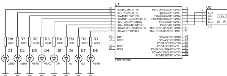
Figura 4.19 | Diagrama de Hardware - indicador luminoso
