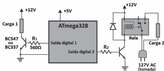
Figura 3.6 | Exemplo de acionamento de dois tipos de cargas digitais
