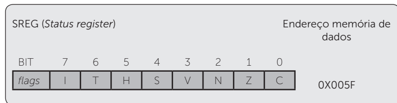
Figura 1.8 | Registrador de status do ATmega328
