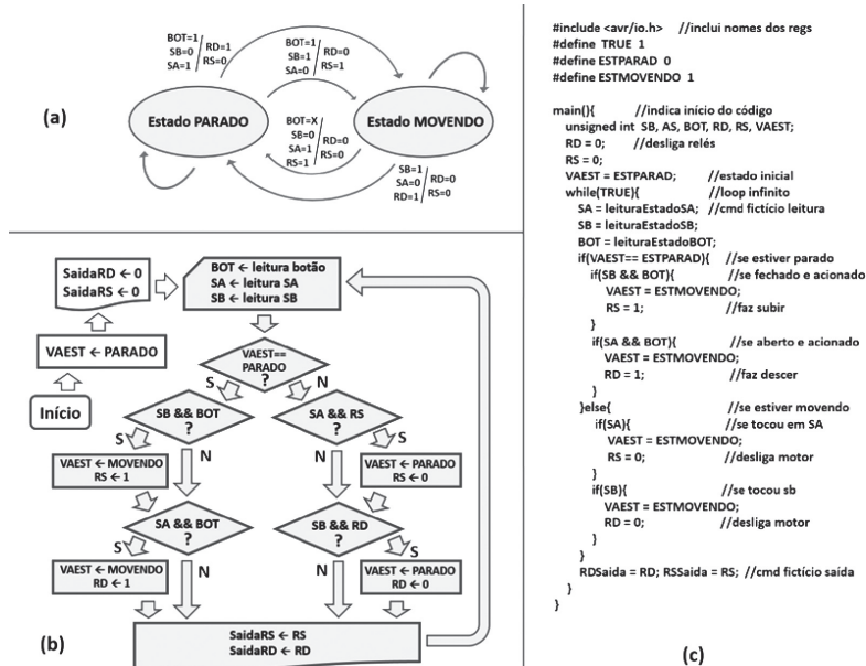
Figura 2.6 | Primeira solução proposta: com MDE: (a) diagrama da MDE; (b) fluxograma; (c) programa
