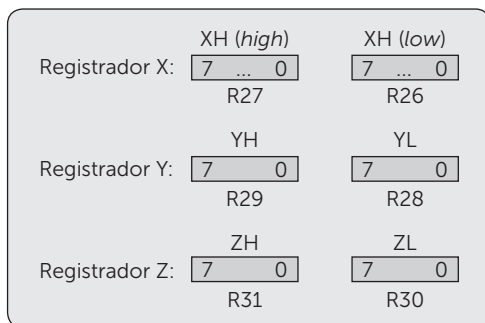
Figura 1.7 | Registradores de 16-bit X, Y e Z
