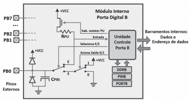
Figura 3.2 | Descrição básica do periférico interno PortB
