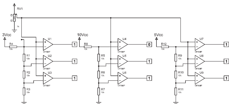
Figura 4.4 | Conversores AD com diferentes tensões de referência
