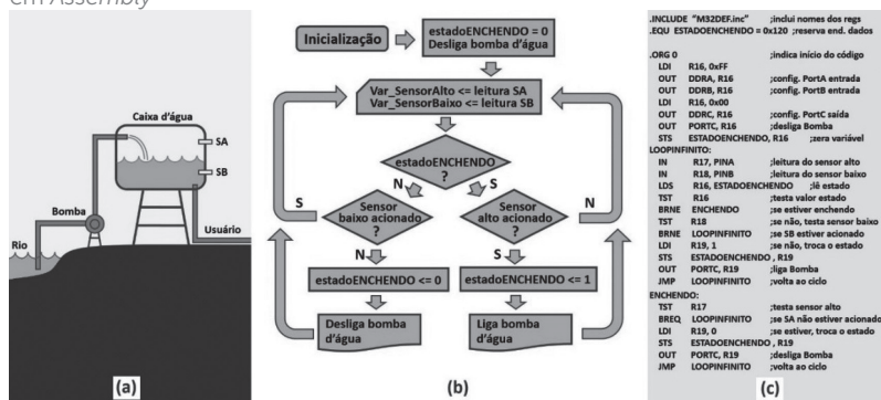
Figura 1.20 | (a) Representação física do problema; (b) fluxograma e (c) programa em Assembly
