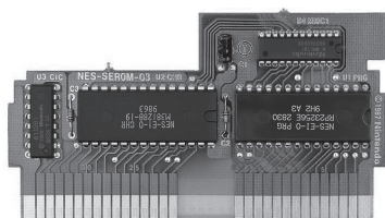
Figura 1.4 | Exemplar de uma placa-cartão (núcleo apenas) para o jogo Tetris
