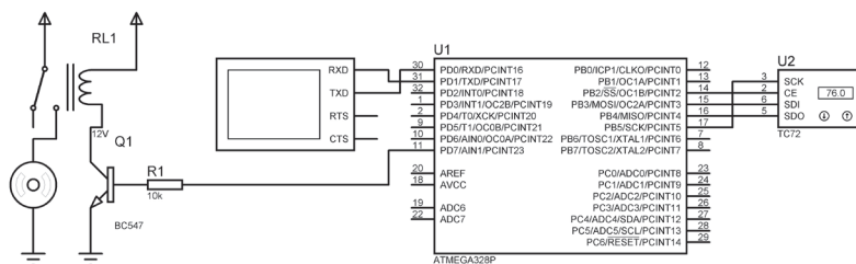
Figura 4.17 | Diagrama de hardware
