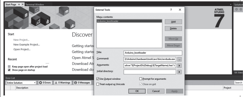
Figura 2.23 | Preenchimento dos campos para o AVRdude
