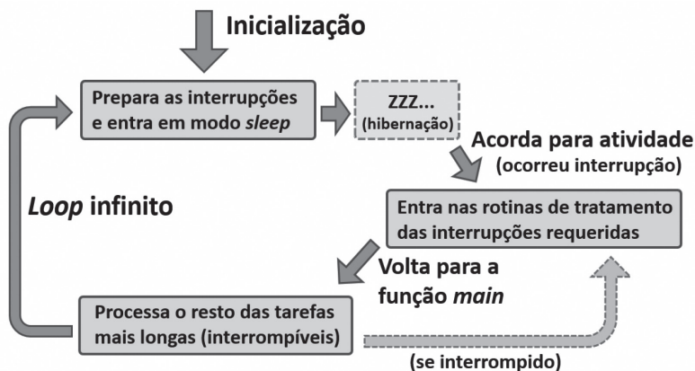
Figura 3.11 | Estrutura básica de um programa embarcado com interrupções e hibernação
