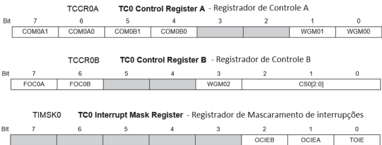
Figura 3.18 | Registradores de configuração do temporizador zero
