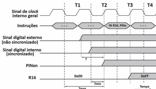
Figura 3.4 | Diagrama temporal da amostragem de um canal digital externo
