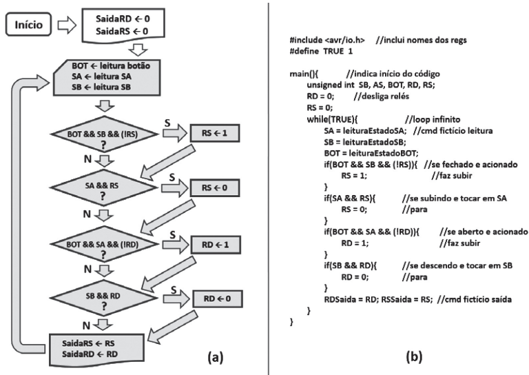
Figura 2.7 | Segunda solução proposta: sem MDE: (a) fluxograma (b) programa
