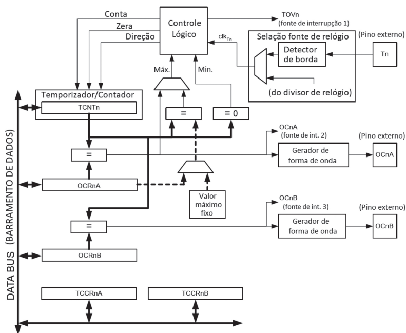
Figura 3.17 | Diagrama interno do módulo temporizador zero do ATmega328
