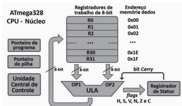
Figura 1.11 | Núcleo do ATmega328
