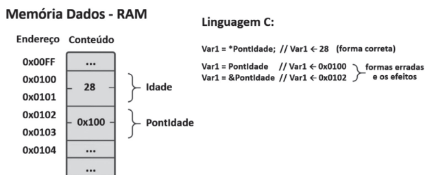
Figura 2.11 | Valores na memória e consequência de comandos em C para o exemplo
