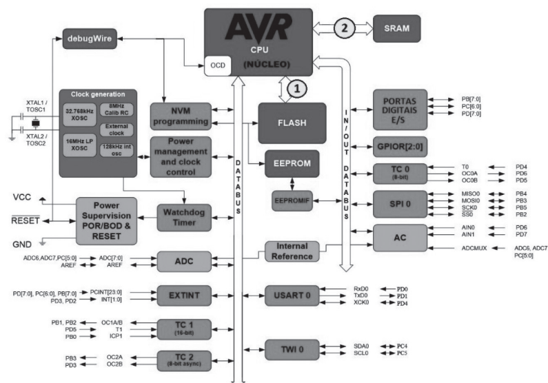
Figura 1.12 | Estrutura interna do microcontrolador ATmega328
