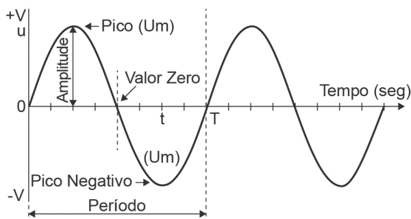
Figura 4.1 | Sinal analógico senoidal
