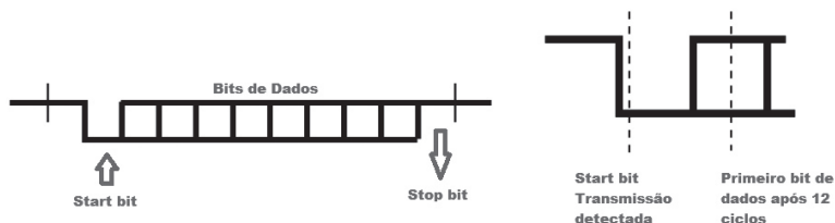
Figura 4.13 | Exemplo de pacote de dados em comunicação assíncrona
