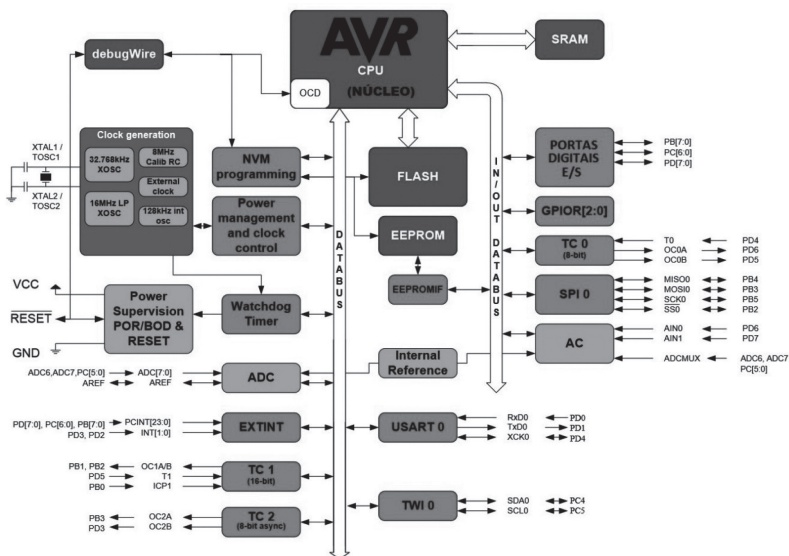
Figura 1.5 | Arquitetura interna do ATmega328
