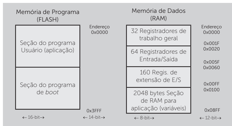
Figura 1.9 | Espaços de memória de programa e de dados do ATmega328
