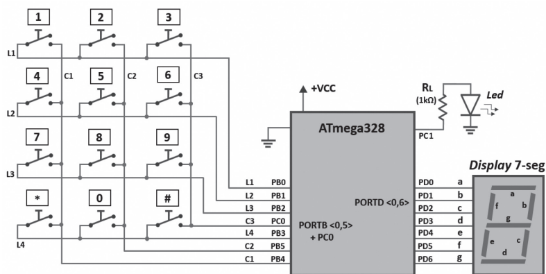
Figura 3.7 | Esquemático proposto como solução do problema (hardware)
