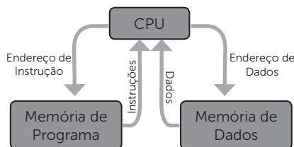
Figura 1.13 | Barramentos da arquitetura Harvard do ATmega328
