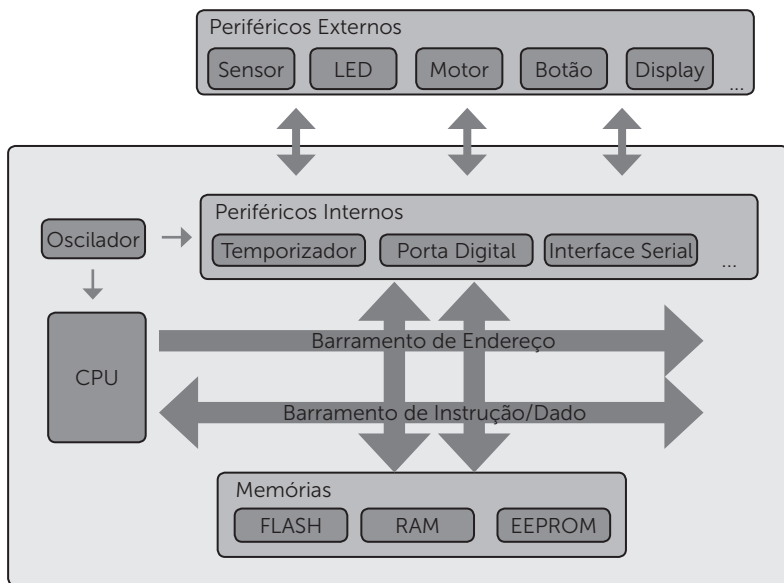
Figura 1.1 | Arquitetura básica de um microcontrolador
