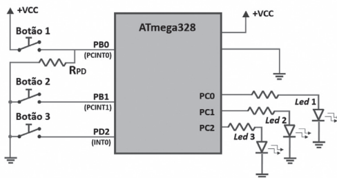
Figura 3.12 | Esquemático para o exemplo
