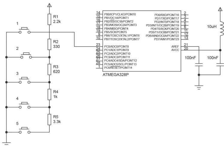
Figura 4.10 | Teclado analógico de 5 teclas
