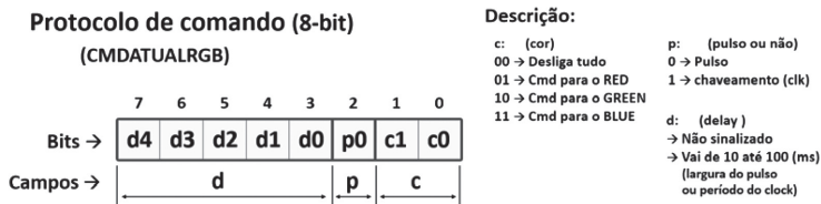
Figura 2.8 | Especificações do protocolo usado em CMDATUALRGB
