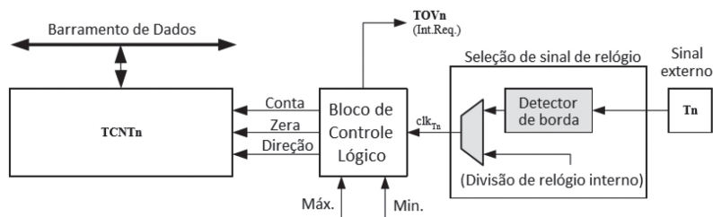
Figura 3.20 | Unidade de contagem do temporizador zero
