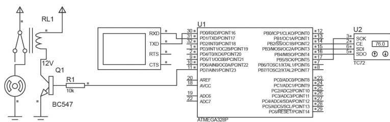
Figura 4.24 | Diagrama de hardware
