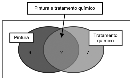
Figura 4.11 | Diagrama de Venn
