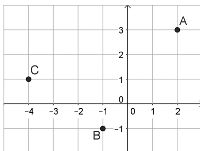
Figura 4.31 | Plano cartesiano com pontos A, B e C
