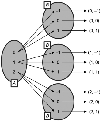
Figura 4.28 | Produto cartesiano de A por B
