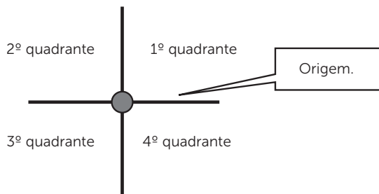
Figura 4.26 | Sistema de eixos determinando os quadrantes
