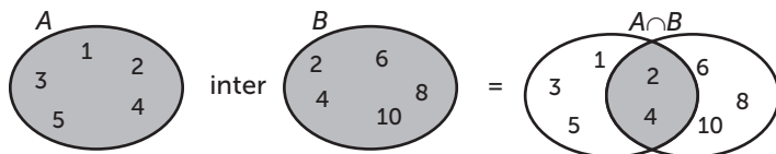
Figura 4.8 | Interseção dos conjuntos A e B
