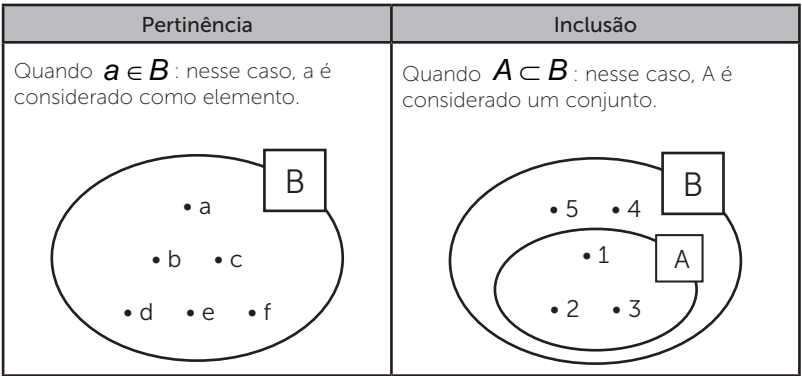
Figura 4.1 | Pertinência e inclusão
