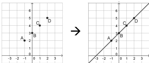
Figura 4.34 | Gráfico de relação
