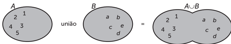
Figura 4.7 | Reunião dos conjuntos A e B
