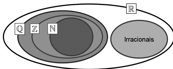
Figura 4.23 | Diagrama de Venn do conjunto dos números reais
