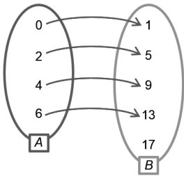
Figura 4.33 | Diagrama de relação
