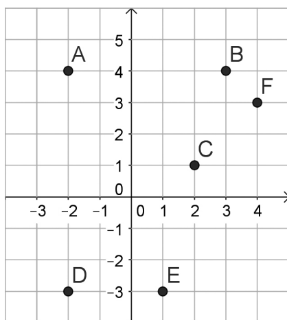
Figura 4.27 | Sistema de eixos com escala
