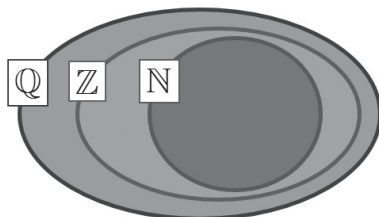
Figura 4.22 | Diagrama de Venn do conjunto dos números racionais
