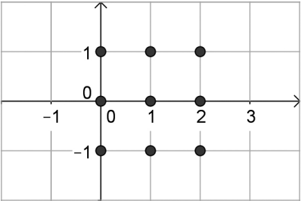
Figura 4.29 | Produto cartesiano de A por B, representado num sistema de eixos
