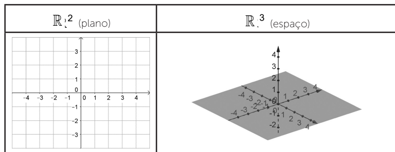
Figura 4.32 | Plano e espaço
