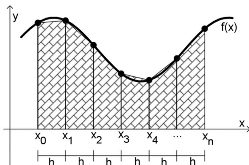
Figura 4.1 | Interpretação gráfica da Regra dos Trapézios
