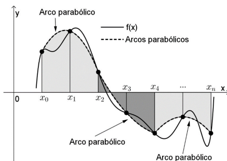
Figura 4.2 | Integração pela Regra de Simpson
