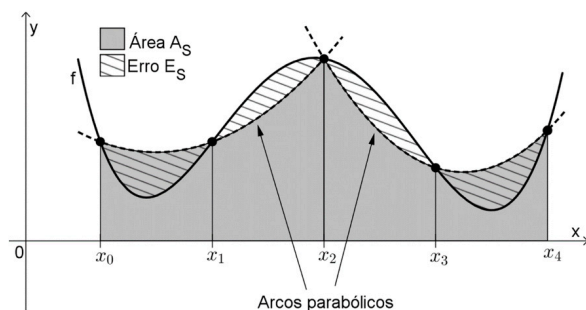
Figura 4.4 | Aproximação para \int_a^b f(x) dx pela Regra de Simpson
