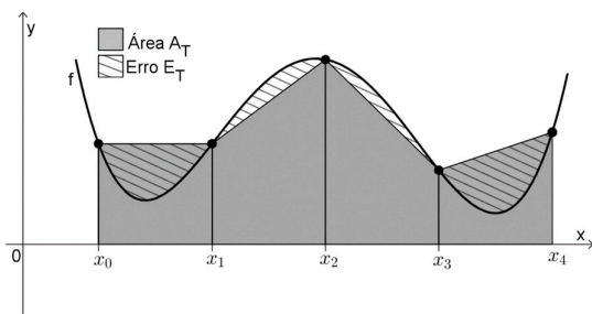
Figura 4.3 | Aproximação para \int_a^b f(x)dx pela Regra dos Trapézios
